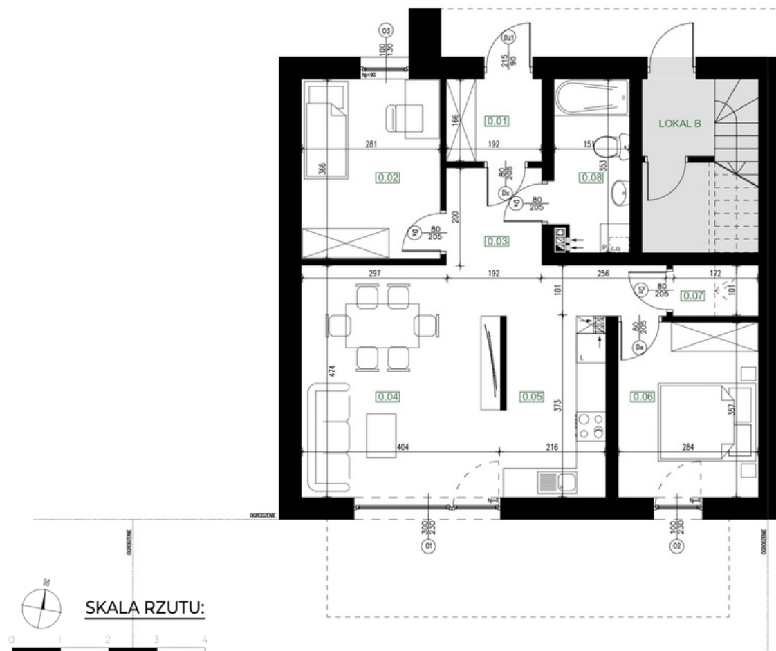
RZUT PARTERU
